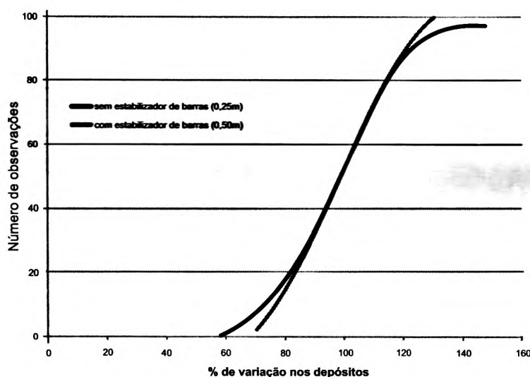
Figura 2. Variações nos depósitos (%) para as aplicações com e sem estabilizador de barra (Dados ajustados).
